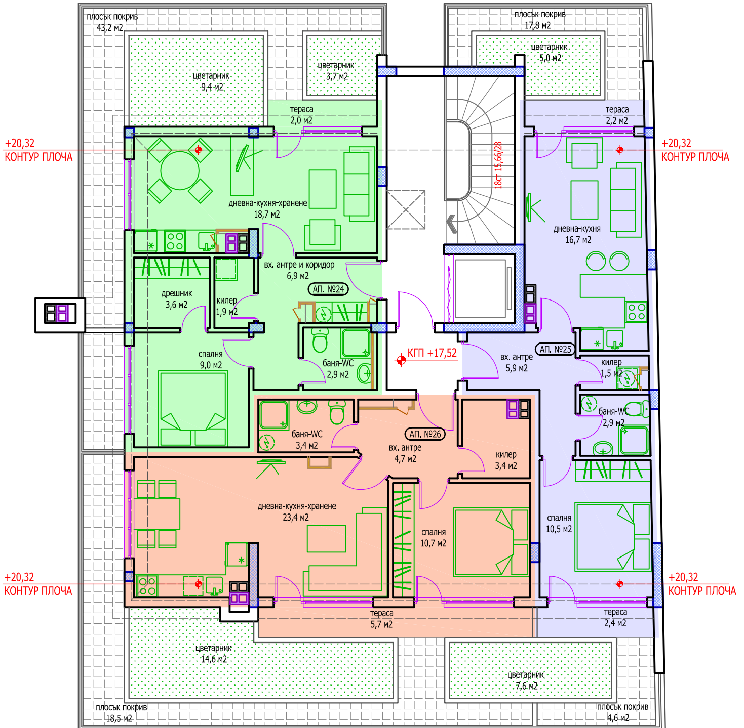
ШЕСТИ ЖИЛИЩЕН ЕТАЖ НА КОТА +17,52 М 1:100
