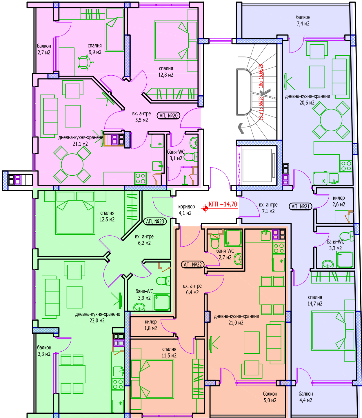
ПЕТИ ЖИЛИЩЕН ЕТАЖ НА КОТА +14,70 М 1:100
