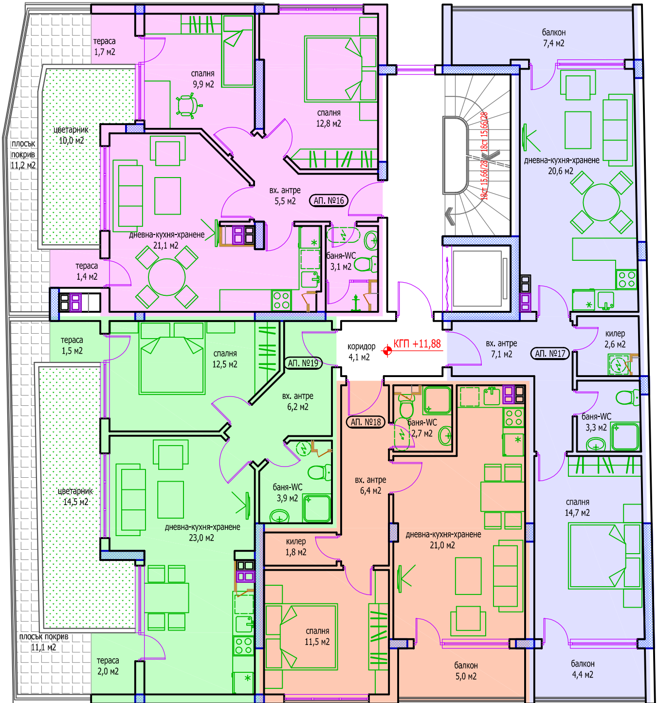
ЧЕТВЪРТИ ЖИЛИЩЕН ЕТАЖ НА КОТА +11,88 М 1:100
