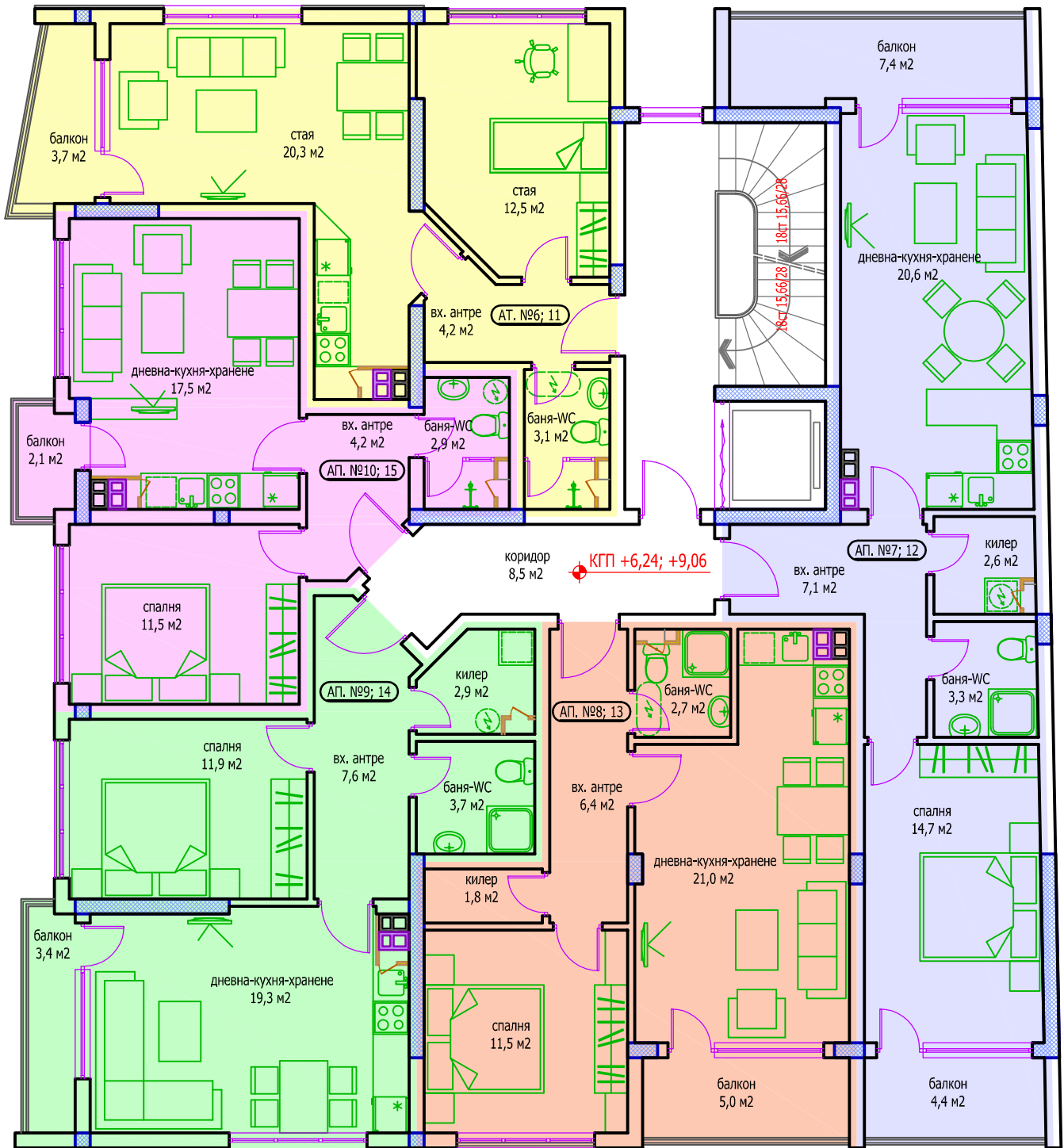
ВТОРИ И ТРЕТИ ЖИЛИЩНИ ЕТАЖИ НА КОТИ +6,24 И +9,06 М 1:100
