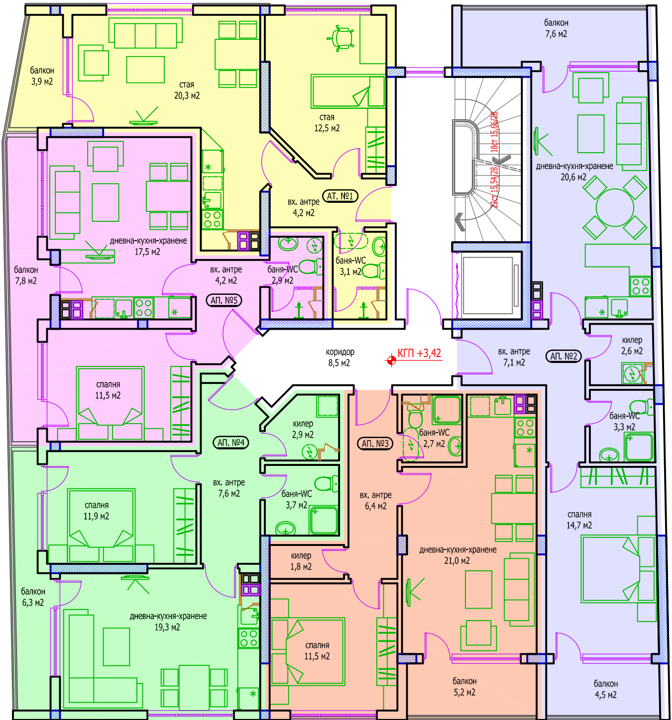
ПЪРВИ ЖИЛИЩЕН ЕТАЖ НА КОТА +3,42 М 1:100
